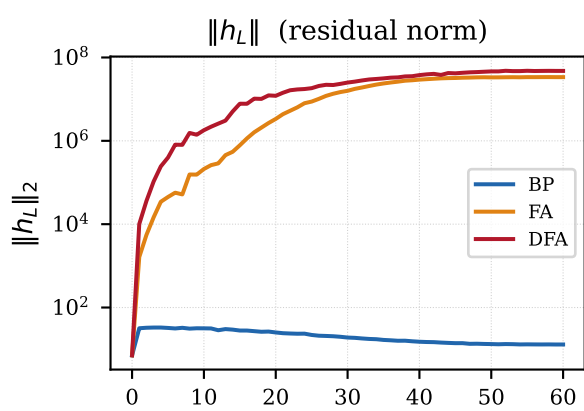
ViT-Mini
