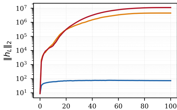
ResMLP no-LN
